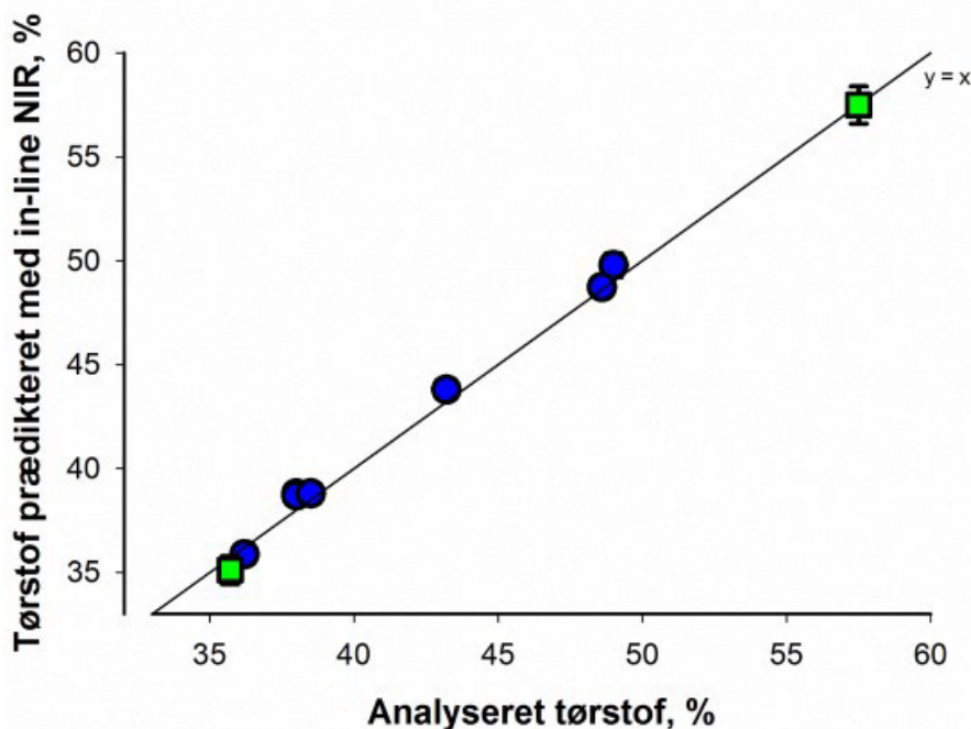
Figur 1. Validering af NIR prædiktioner af tørstof ved scanning på fuldfoderblander (JF-Stoll VM-22 blander, Dinamica Generale NIR). Blå cirkler indikerer scanning af slut-mix og grønne firkanter indikerer scanning af mellem-mix. Hvert punkt angiver gennemsnit af 5 scan-sekvenser med angivelse af standardafvigelsen (ikke alle standardafvigelser er synlige fordi de er mindre end symbolet).
